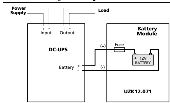
Fig. 9-1 Wiring scheme
