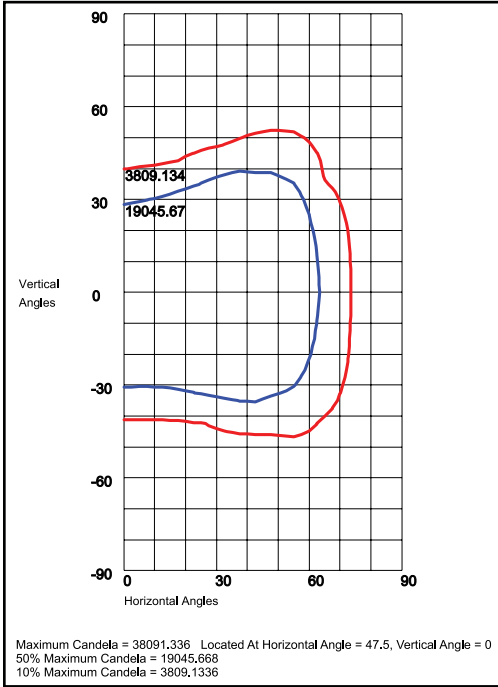
KH55QA2X256U5KC 130°H x 70°V, NEMA 7H x 5V
