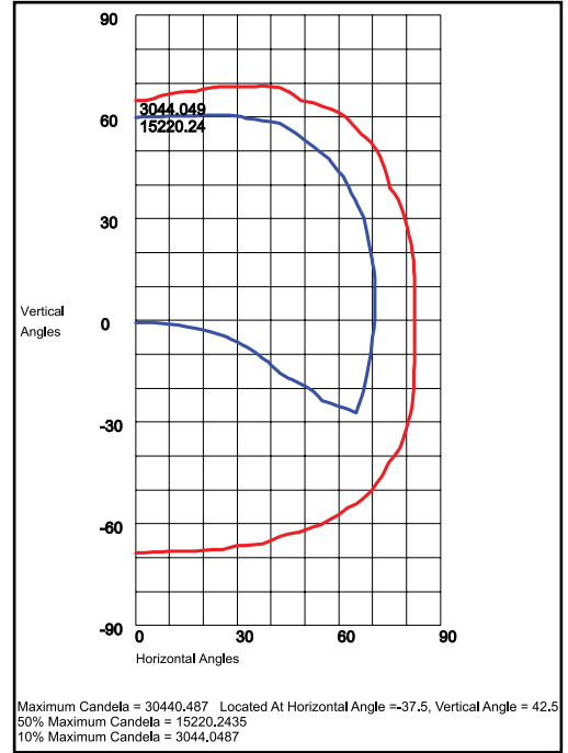
KH55QC2X256U5KC 120°H x 70°V, NEMA 7H x 7V
