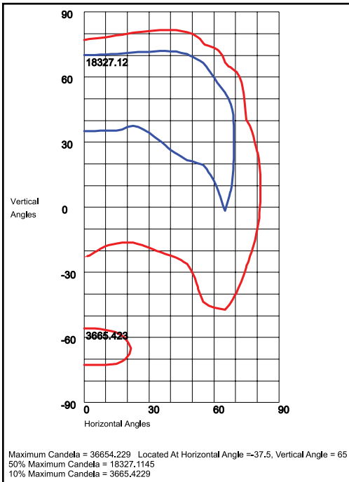
KH55QD2X256U5KC 110°H x 30°V, NEMA 6H x 5V
